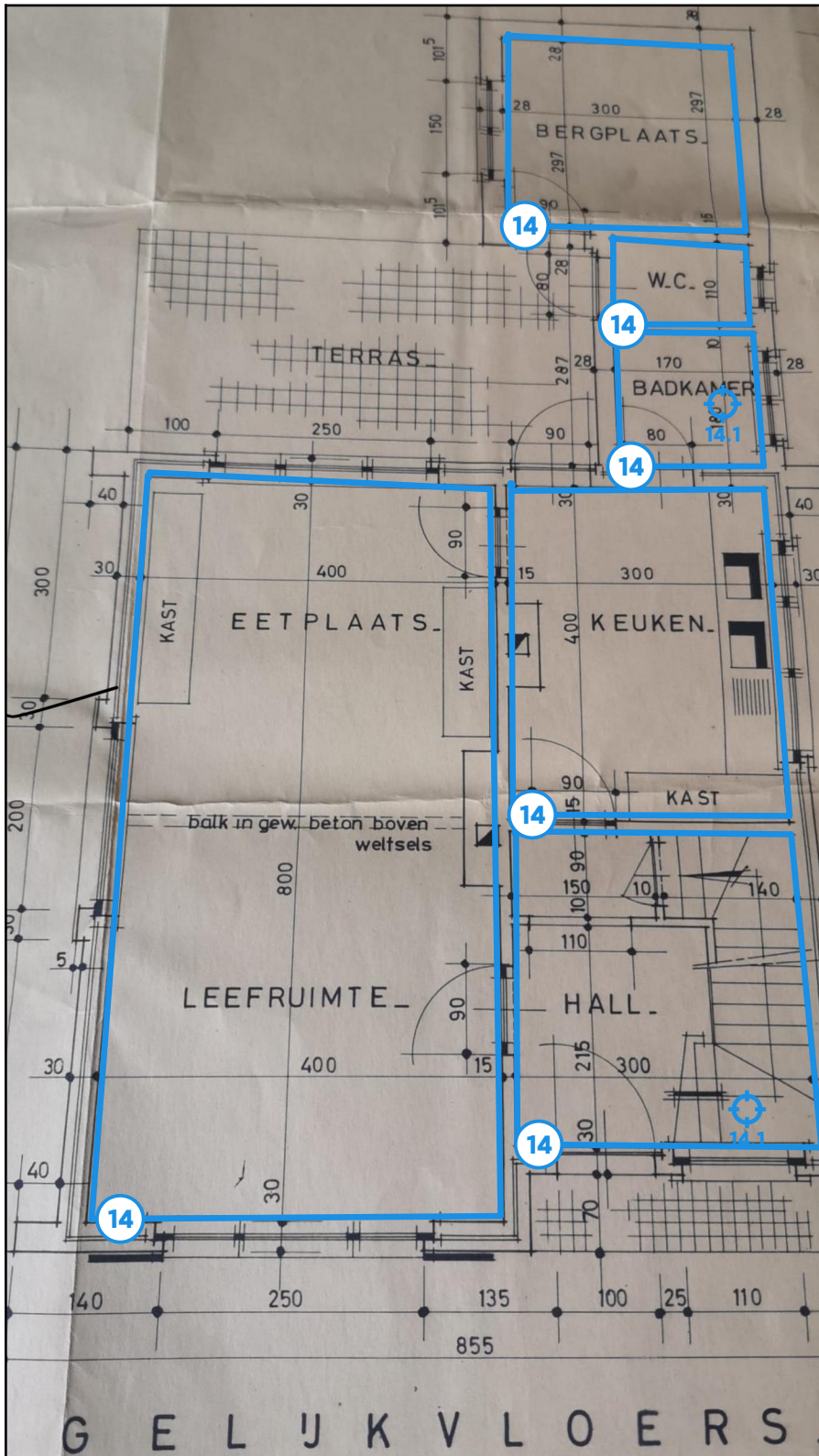
Legende van plan 1.2: Gelijkvloers pleisterwerk muren
